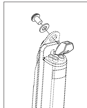
UT-PU020 Adattatore per installazione rovesciata PU EPS V2
